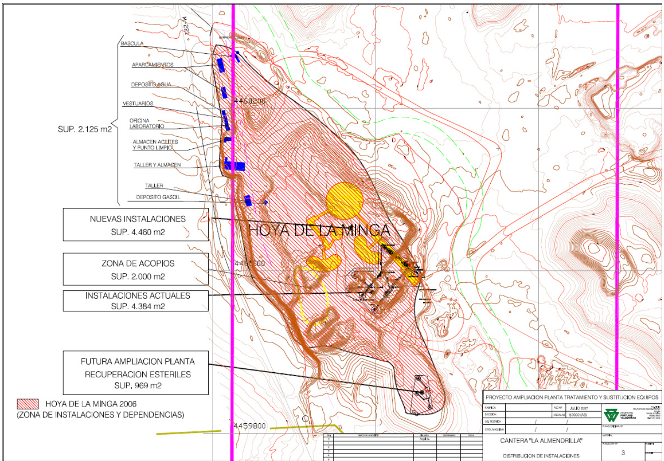
Figura 16. Plano de detalle de ubicación de la planta y la superficie que ocupa cada una de las instalaciones.
