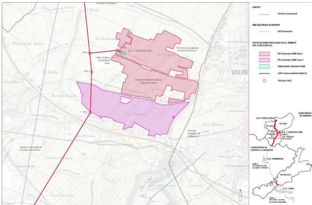
PLANTA POR TRAMOS. PLANTA FOTOVOLTAICA ENVATIOS XXIII. HOJA 3 DE 5.
