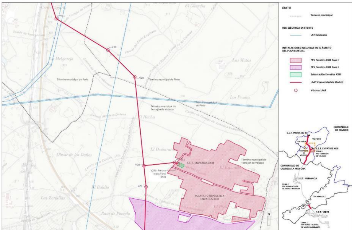
PLANTA POR TRAMOS. LÍNEA AÉREA DE ALTA TENSIÓN ENVATIOS XXIII. HOJA 2 DE 5.
