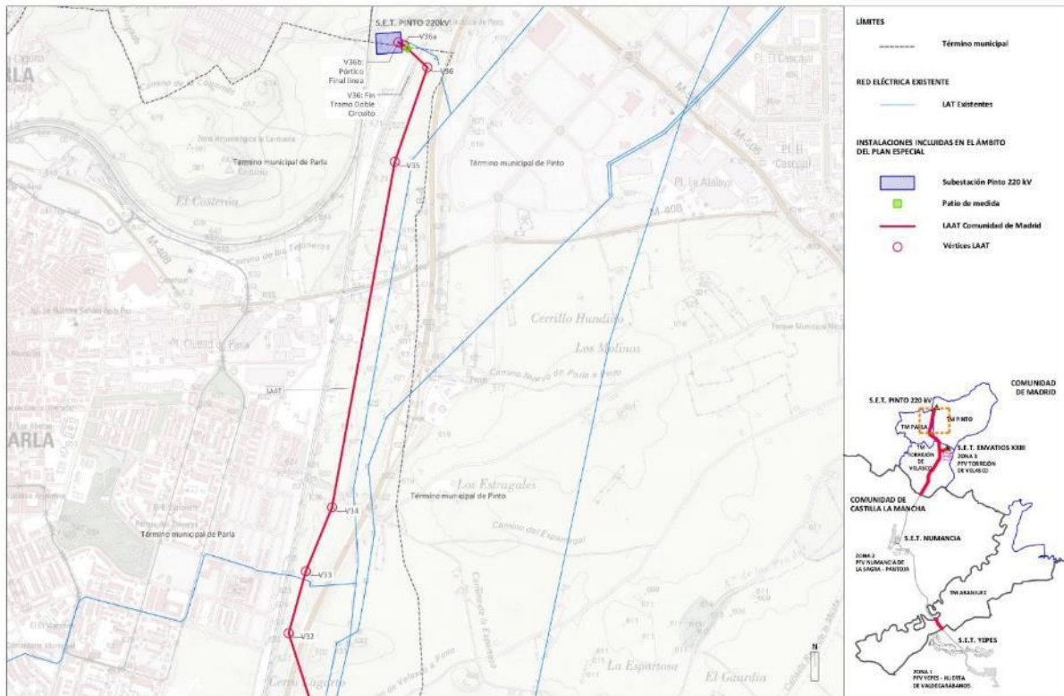
PLANTA POR TRAMOS. LÍNEA AÉREA DE ALTA TENSIÓN ENVATIOS XXIII. HOJA 1 DE 5.
