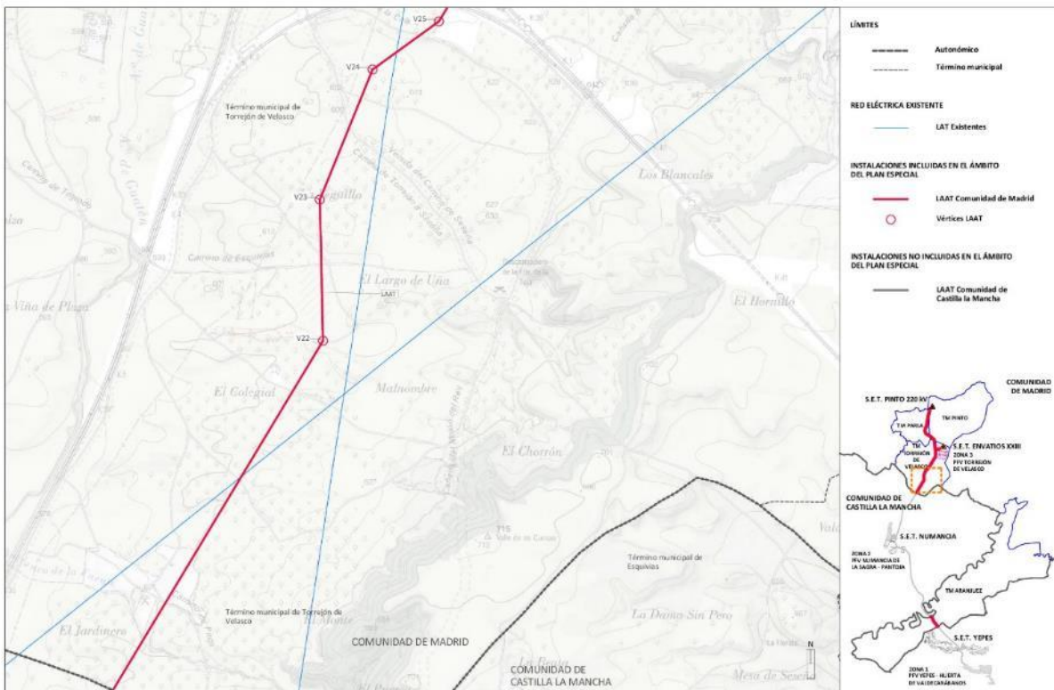
PLANTA POR TRAMOS. LÍNEA AÉREA DE ALTA TENSIÓN ENVATIOS XXIII. HOJA 4 DE 5.
