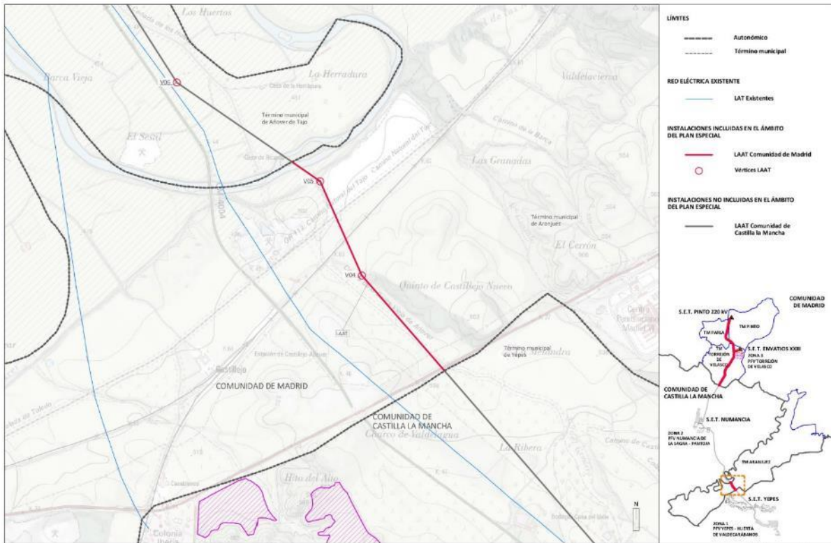
PLANTA POR TRAMOS. LÍNEA AÉREA DE ALTA TENSIÓN ENVATIOS XXIII. HOJA 5 DE 5.
