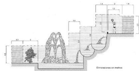
Figura 5. Volúmenes de protección en fuentes
