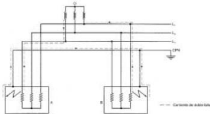
Figura 7. Corriente de segundo defecto en el esquema IT con masa conectada a la misma toma de tierra y neutro no distribuido.
