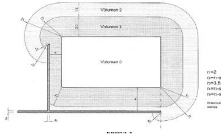
Figura 4. Volúmenes de protección en piscinas con paredes
