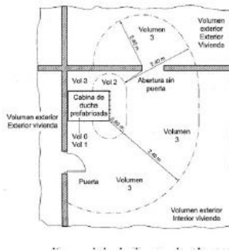
Figura 7 – CABINA DE DUCHA PREFABRICADA
