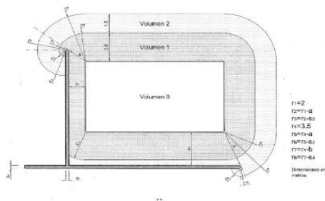
Figura 4. Volúmenes de protección en piscinas con paredes
