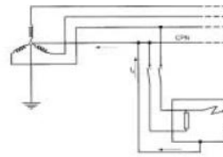
Figura 2. Esquema TN-C.
