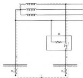
Figura 4 Esquema TT
