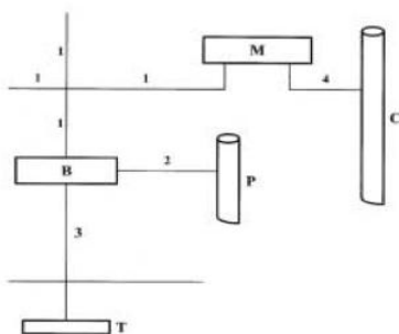
Figura 1. Representación esquemática de un circuito de puesta a tierra
