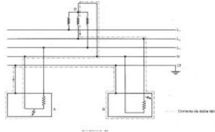
Figura 8. Corriente de segundo defecto en el esquema IT con masa conectada a la misma toma de tierra y neutro distribuido.
