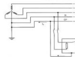
Figura 3. Esquema TN-S.
