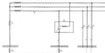
Figura 6. Esquema IT unido a tierra por impedancia Z_n y con las puestas a tierra de la alimentación y de las masas separadas
