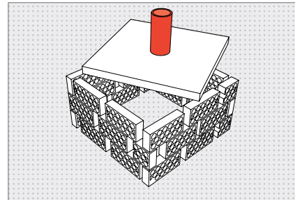
1 vaciado 2 conducto de extracción
