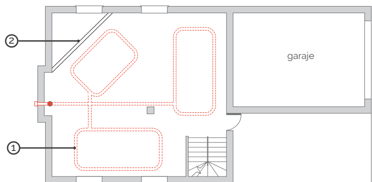
Figura 3 - Distribución de la red de tubos perforados
