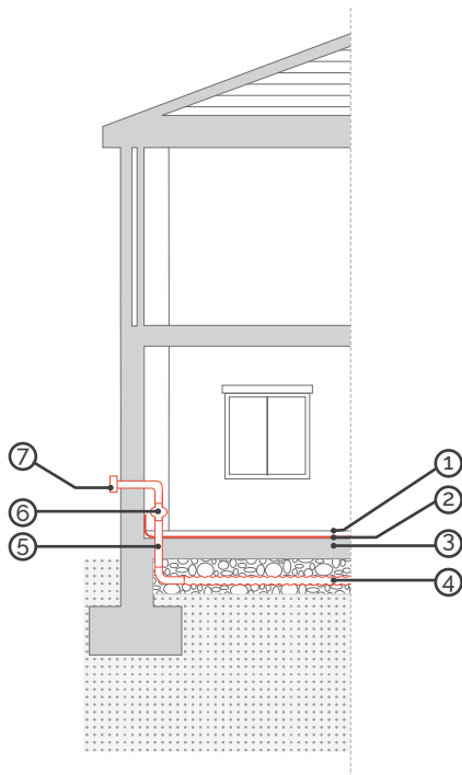
Figura 2 - Sección de la solución
