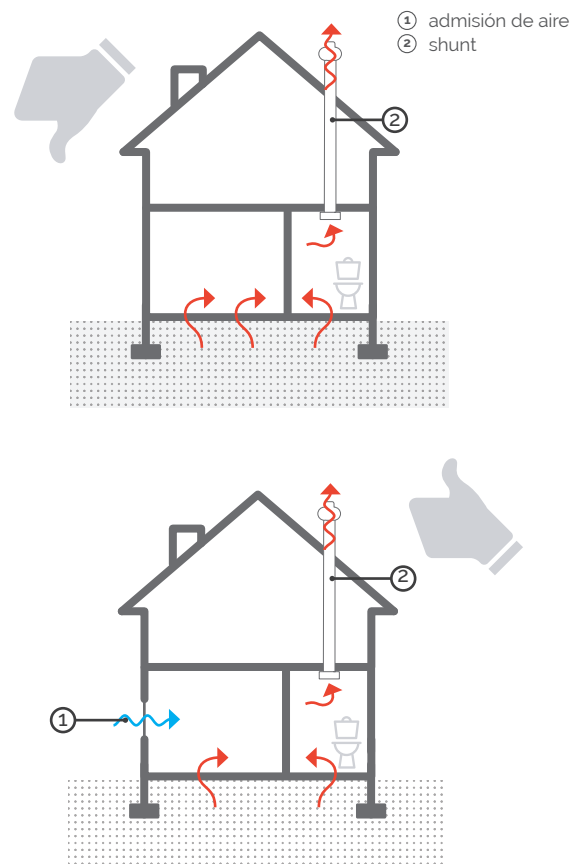
Figura 6 - Sistema de ventilación sin (izda.) y con (drcha.) abertura de admisión de aire exterior
