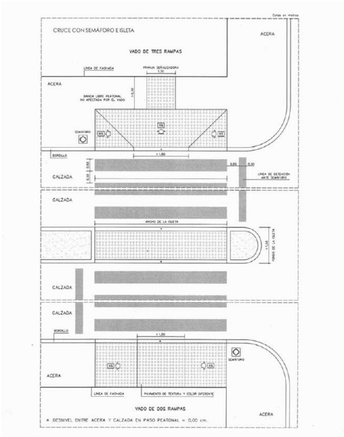
GRÁFICO 5. VADOS
