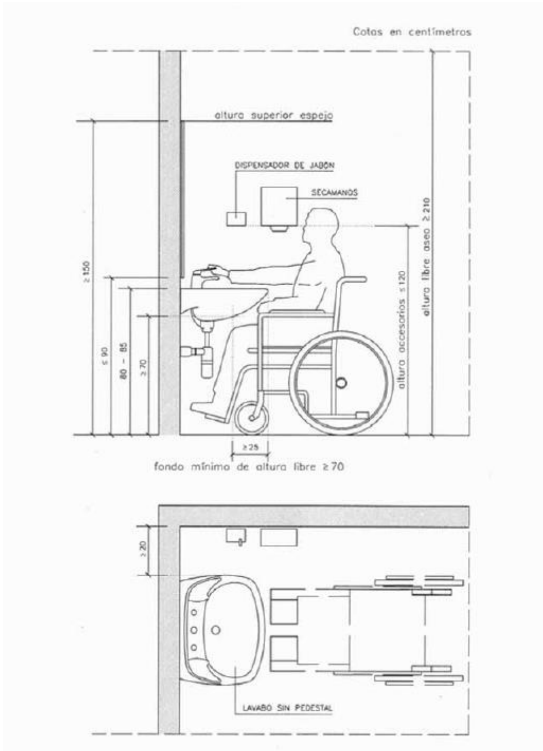
GRÁFICO 13. LAVABO ACCESIBLE
