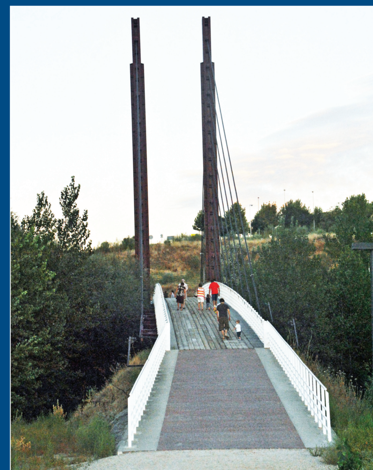
Pasarela peatonal.
