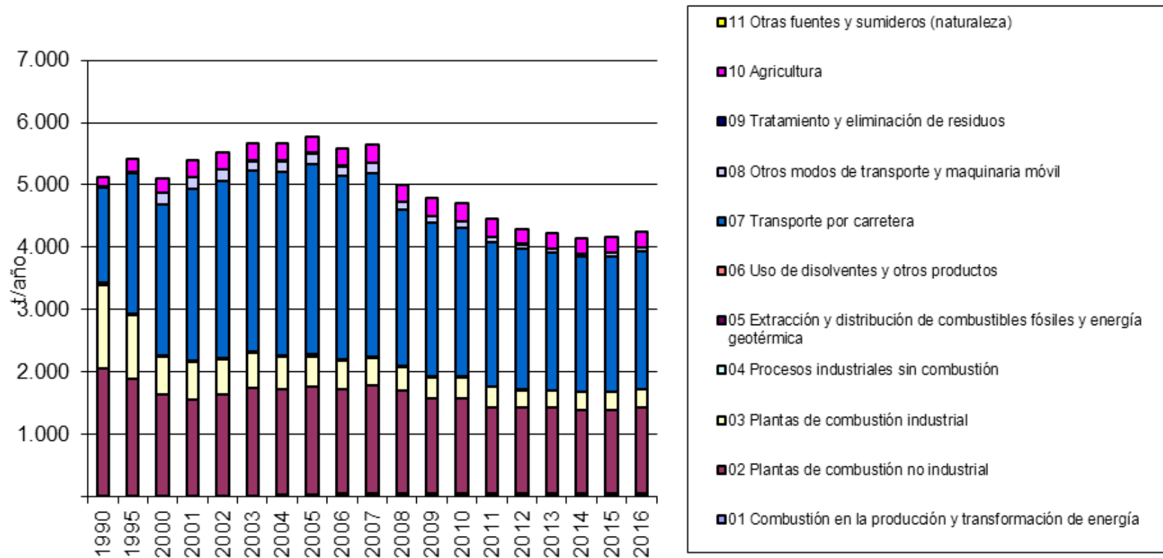
Figura 22. Evolución de las emisiones de PM 10 (t/año)
