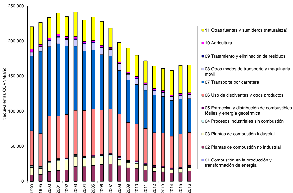
Figura 29. Evolución de la contribución a la formación de ozono troposférico de las emisiones de la Comunidad de Madrid (t equivalentes de COVNM/año)
