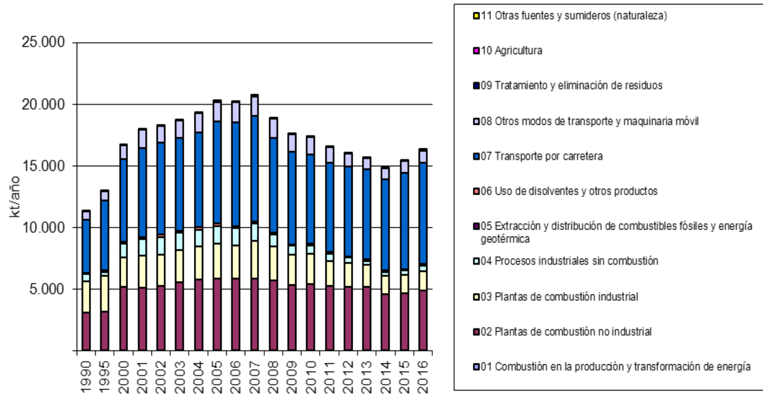
Figura 6. Evolución de las emisiones de CO 2 (kt/año)
