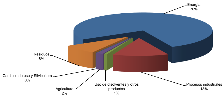
Figura 37. Emisiones de GEIs por fuente de emisión en la Comunidad de Madrid en el año 2017
