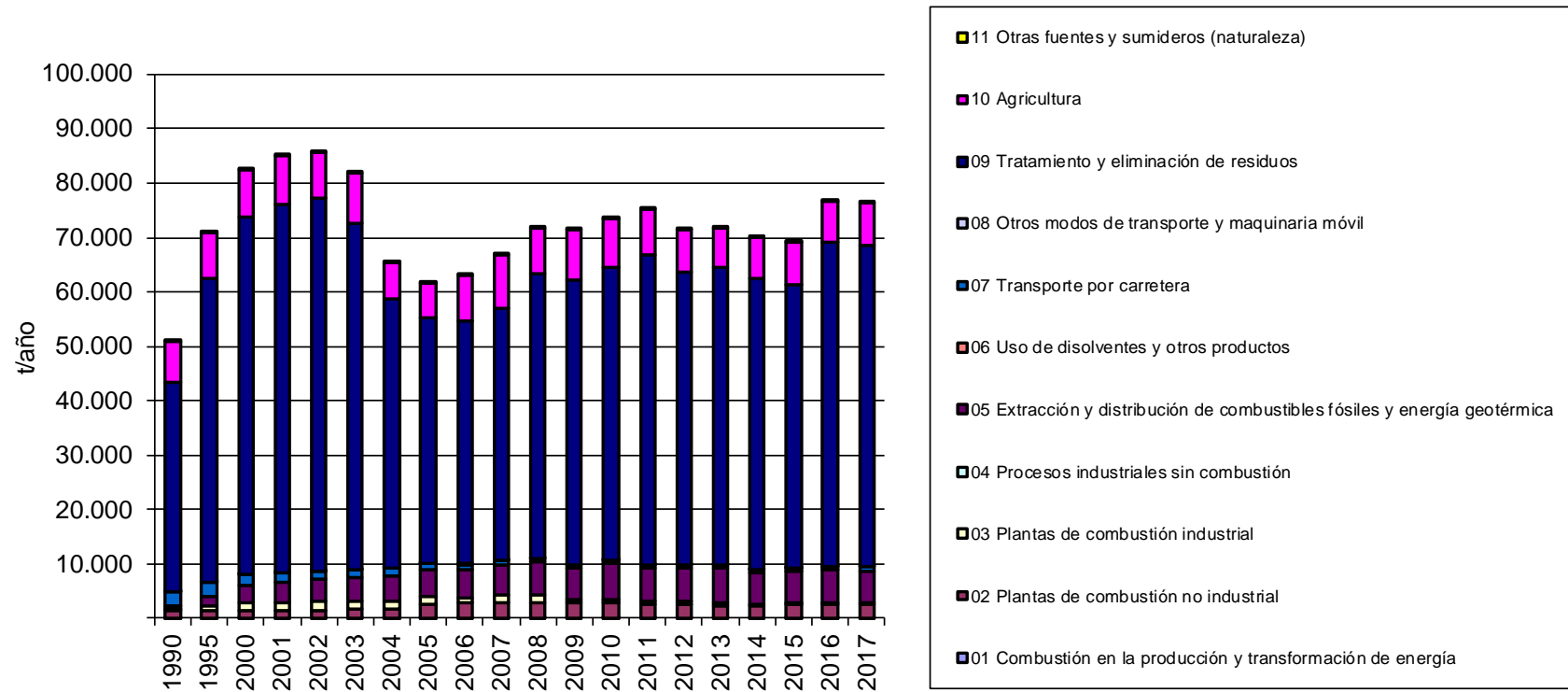
Figura 4. Evolución de las emisiones de CH 4 (t/año)
