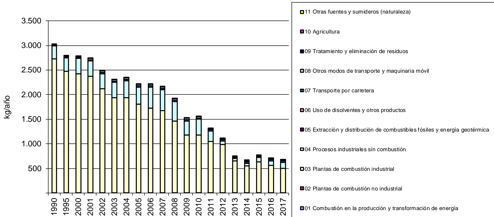
Figura 17. Evolución de las emisiones de Ni (kg/año)
