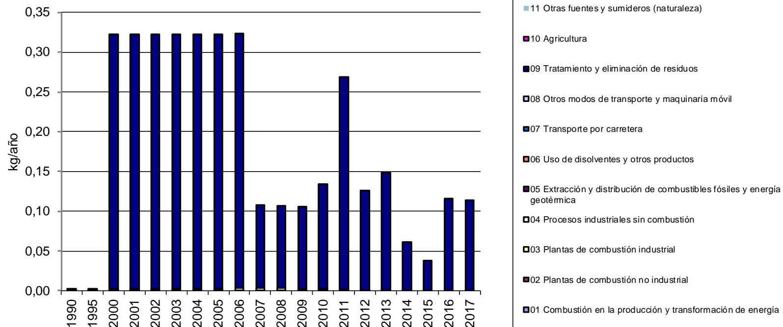
Figura 26. Evolución de las emisiones de Hexaclorobenceno (HCB) (kg/año)
