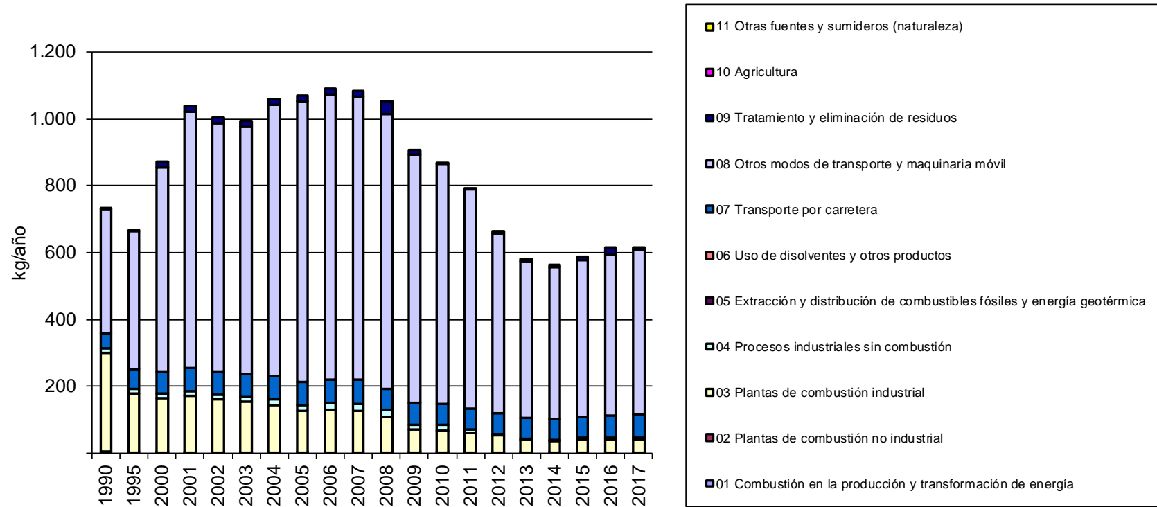
Figura 15. Evolución de las emisiones de Cu (kg/año)
