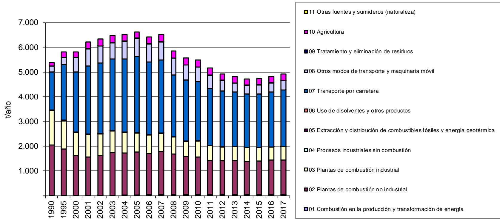
Figura 22. Evolución de las emisiones de PM 10 (t/año)
