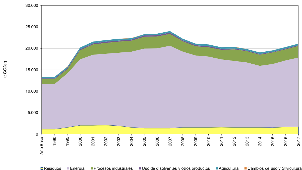
Figura 34. Emisiones de GEI de los diferentes sectores analizados desde el año base hasta el año 2017 (ktCO 2 eq)
