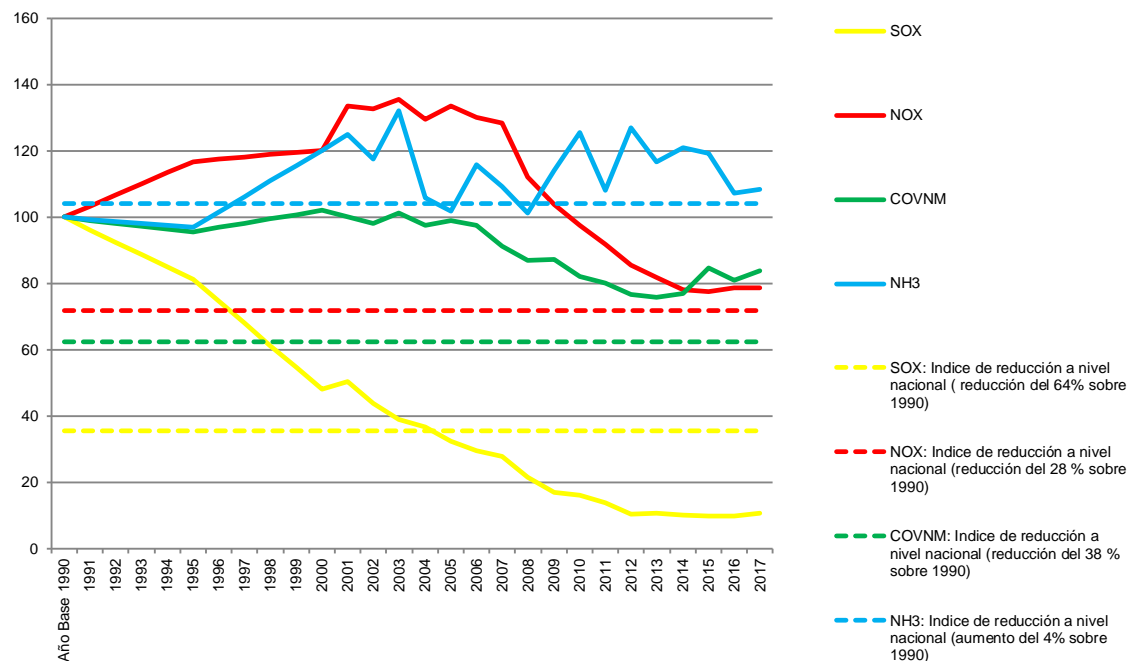
Figura 31. Evolución de las emisiones en la Comunidad de Madrid de aquellos contaminantes para los que se han establecido techos nacionales de emisión mediante la Directiva 81/2001 (emisiones del año 1990=100)
