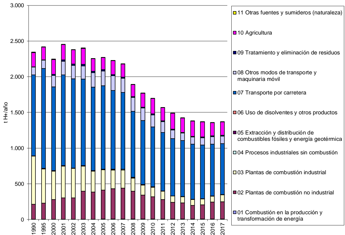
Figura 30. Evolución de la contribución a la acidificación de las emisiones atmosféricas de la Comunidad de Madrid (t de hidrogeniones / año)
