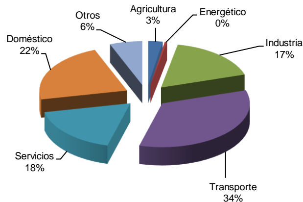
Figura 39. Distribución sectorial de las emisiones totales (directas+indirectas) de GEI de la Comunidad de Madrid en el año 2017
