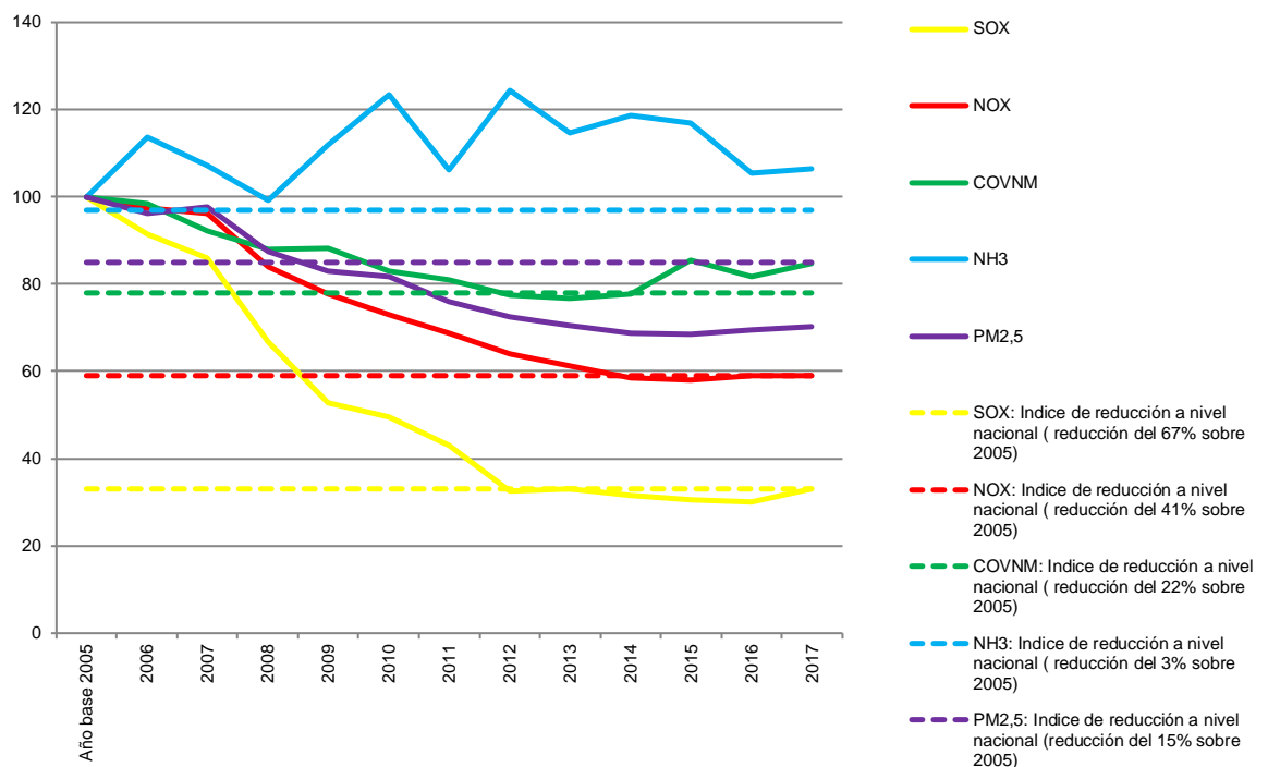
Figura 32. Evolución de las emisiones en la Comunidad de Madrid de aquellos contaminantes para los que se han establecido techos nacionales de emisión mediante la Directiva 2016/2284 (emisiones del año 2005=100)
