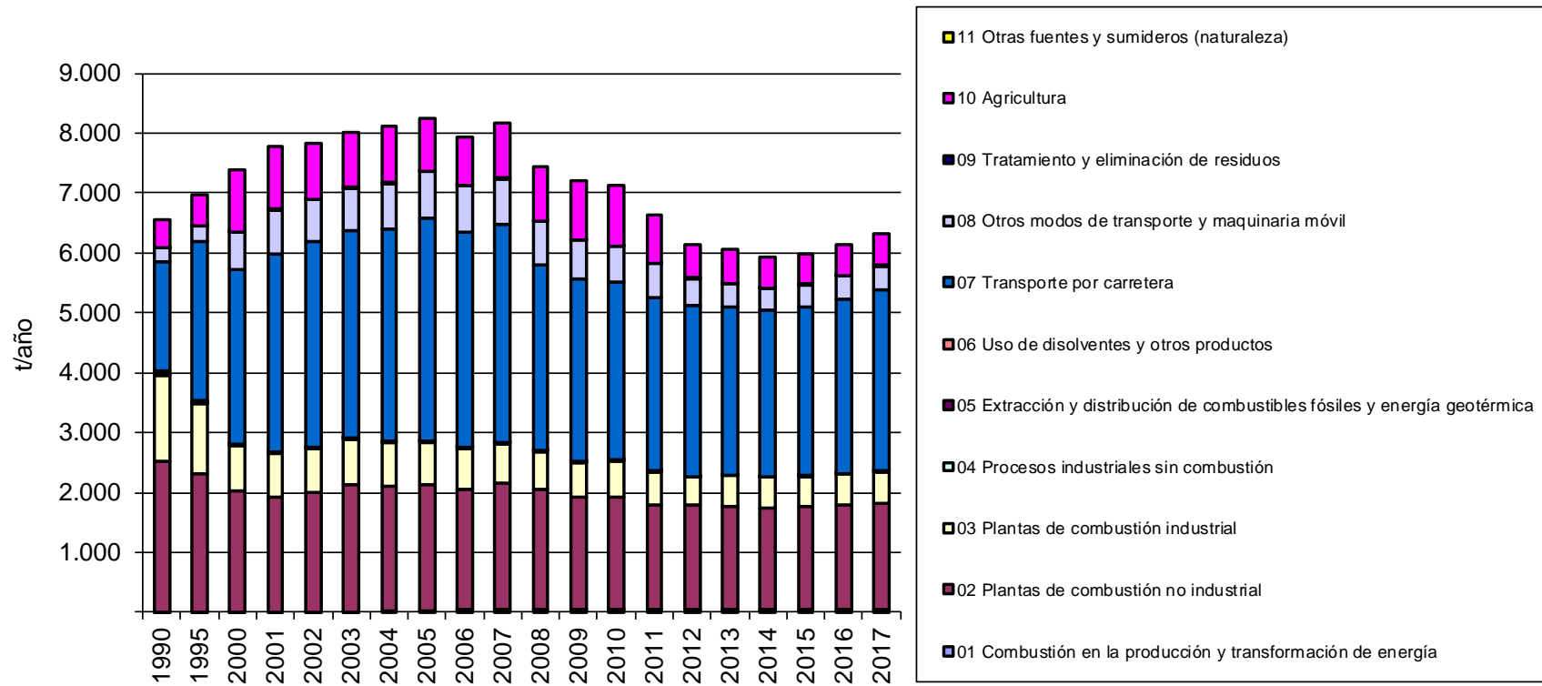
Figura 23. Evolución de las emisiones de PST (t/año)
