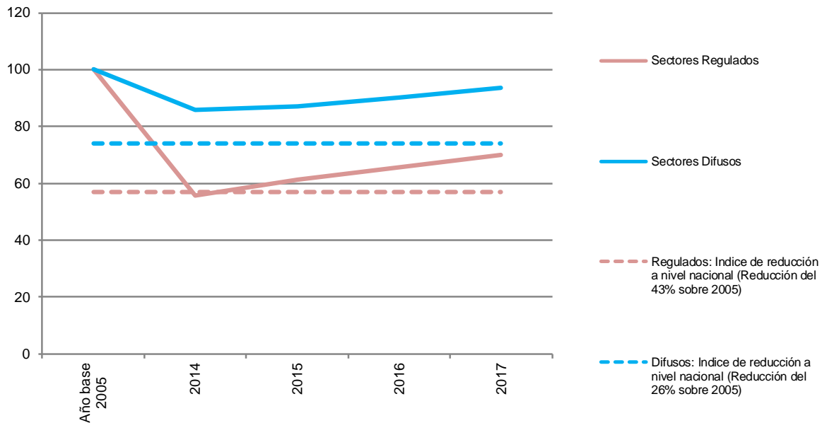
Figura 35. Evolución de las emisiones GEI en la Comunidad de Madrid en relación con los objetivos establecidos a nivel nacional para el 2030 (emisiones del año 2005=100)
