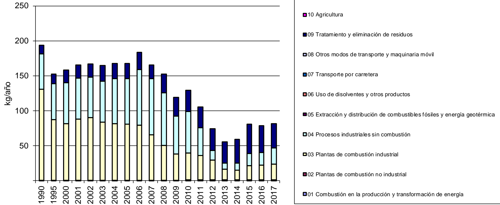
Figura 16. Evolución de las emisiones de Hg (kg/año)
