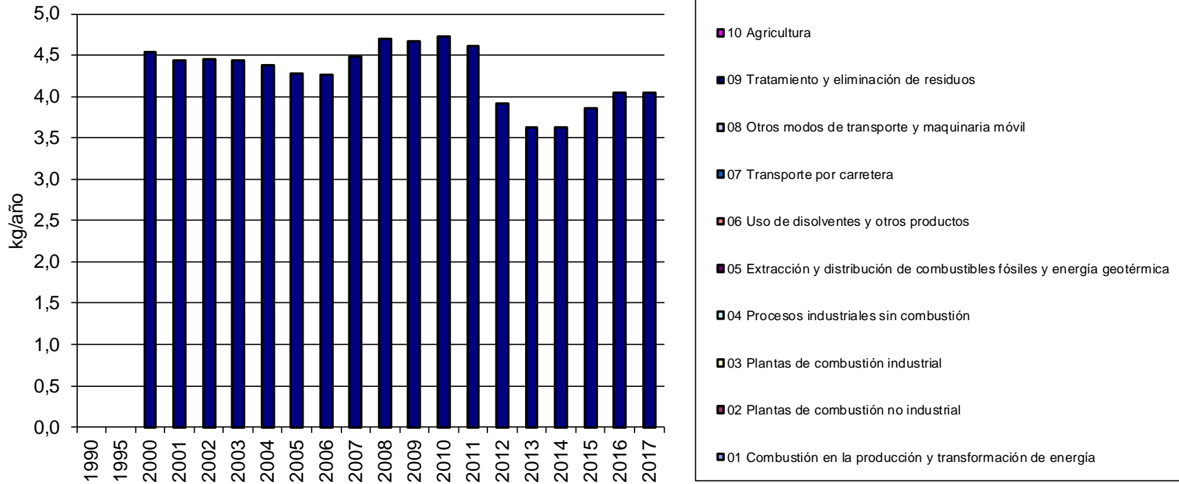
Figura 25. Evolución de las emisiones de Pentaclorofenol (PCP) (kg/año)
