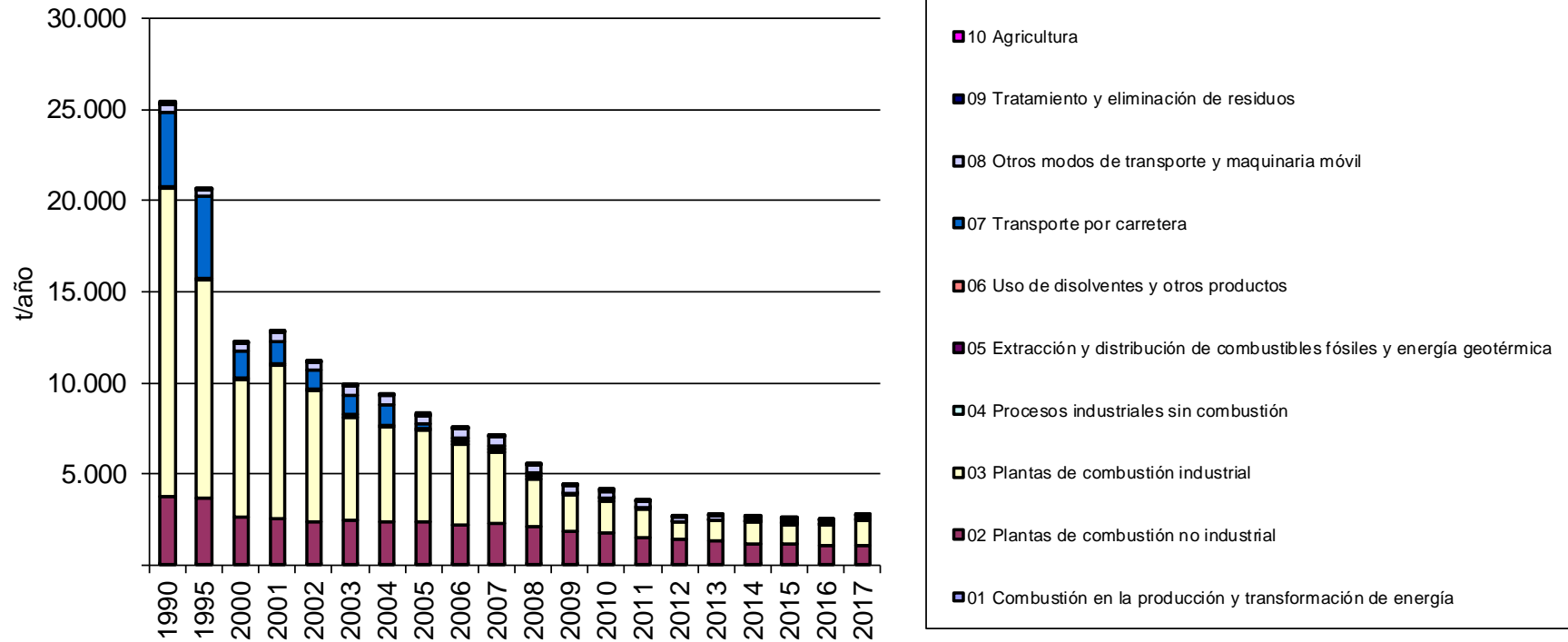
Figura 1. Evolución de las emisiones de SOx (t/año)
