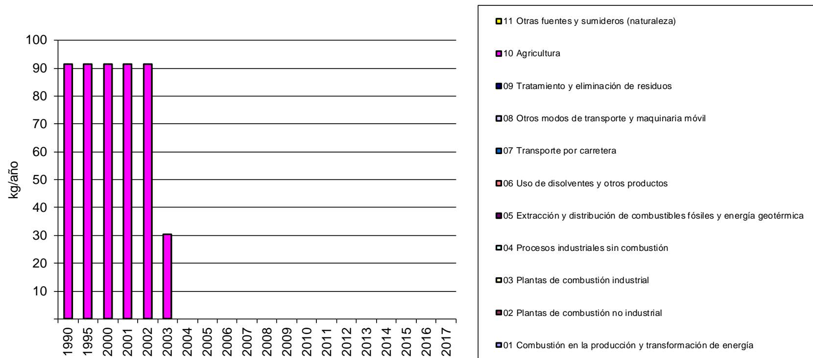
Figura 24. Evolución de las emisiones de Hexaclorociclohexano (HCH) (kg/año)
