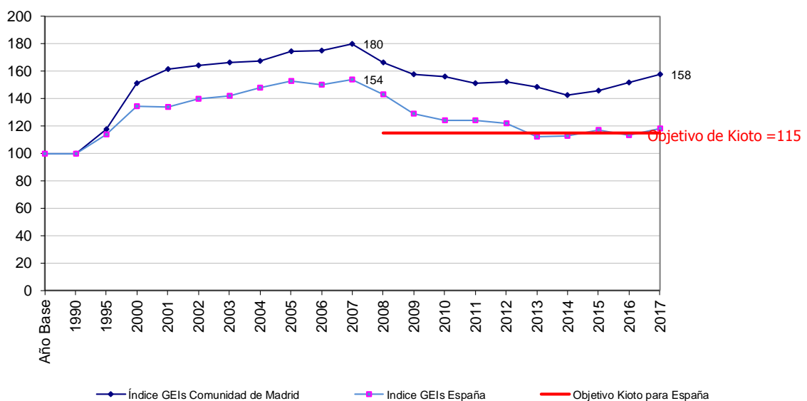
Figura 33. Índice de evolución de las emisiones de gases de efecto invernadero en la Comunidad de Madrid, en la Unión Europea y en España (año base 1990=100)
