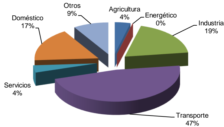
Figura 38. Distribución sectorial de las emisiones directas de GEI de la Comunidad de Madrid en el año 2017
