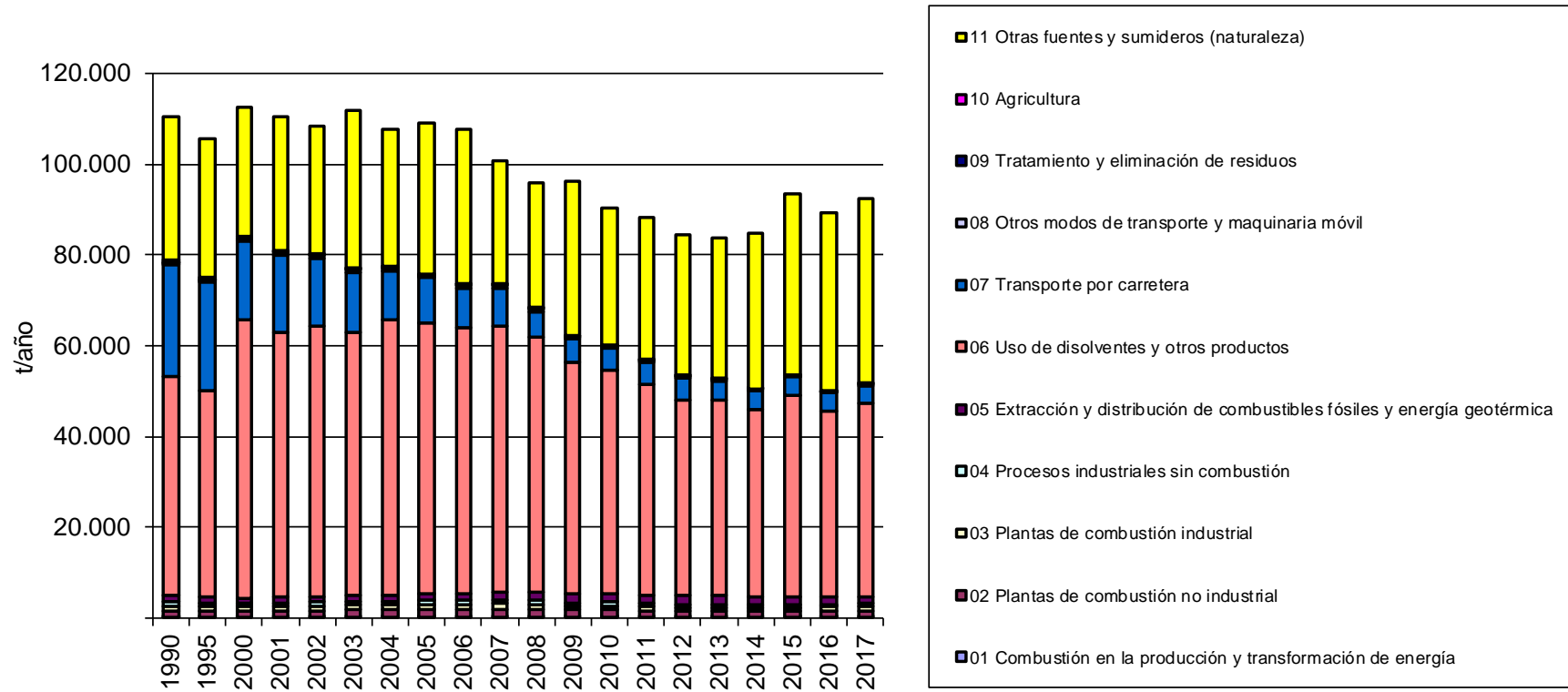
Figura 3. Evolución de las emisiones de COVsNM (t/año)
