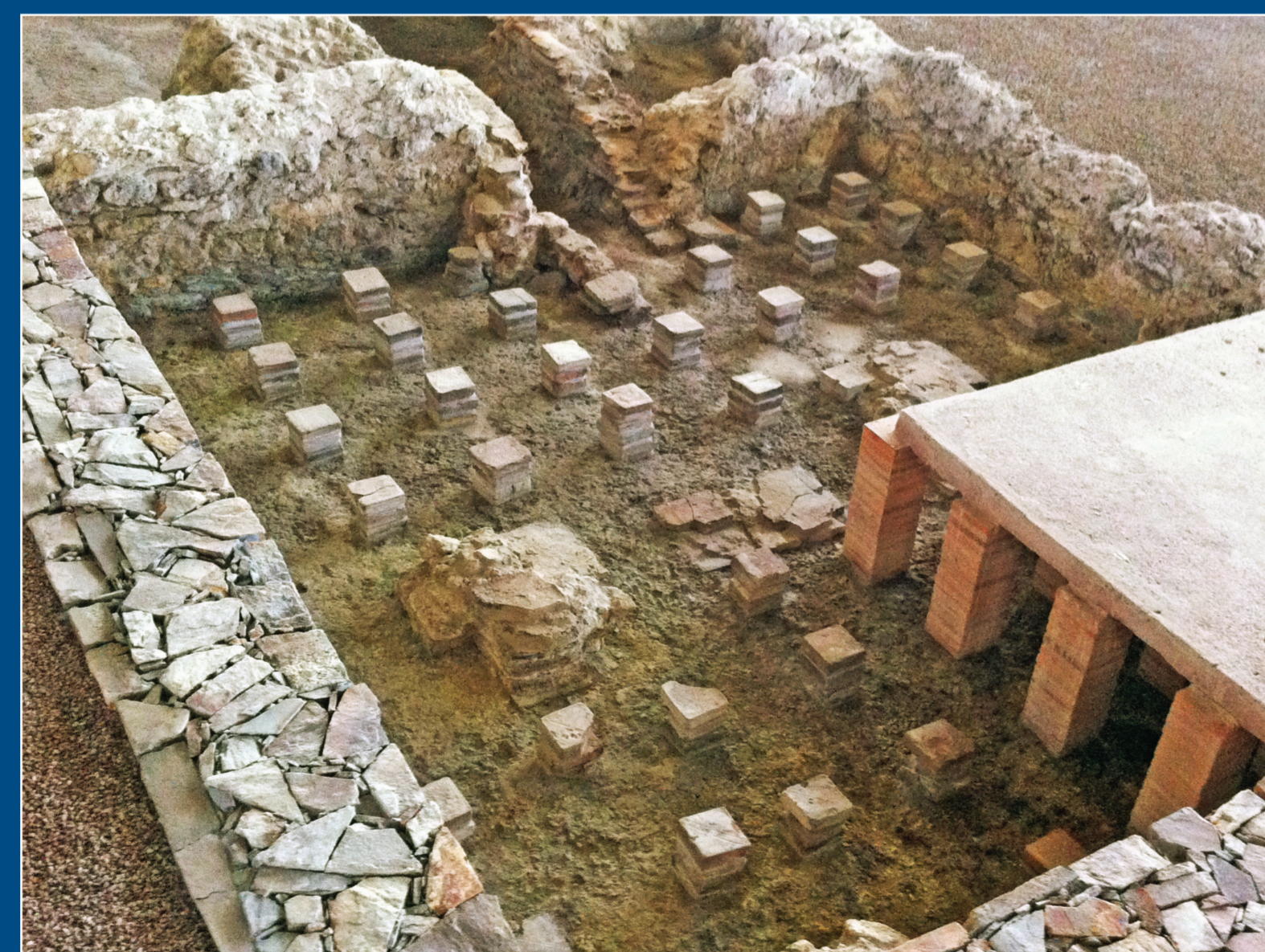
Termas romanas de la villa de La Olmeda (Valladolid).
