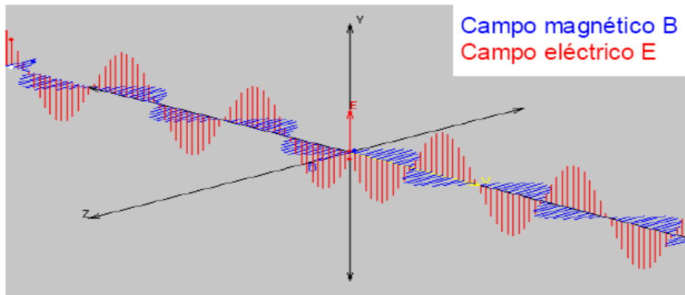
Figura 8.5.2.2.2 Campo eléctrico y magnético (Fuente: CEDEX)
