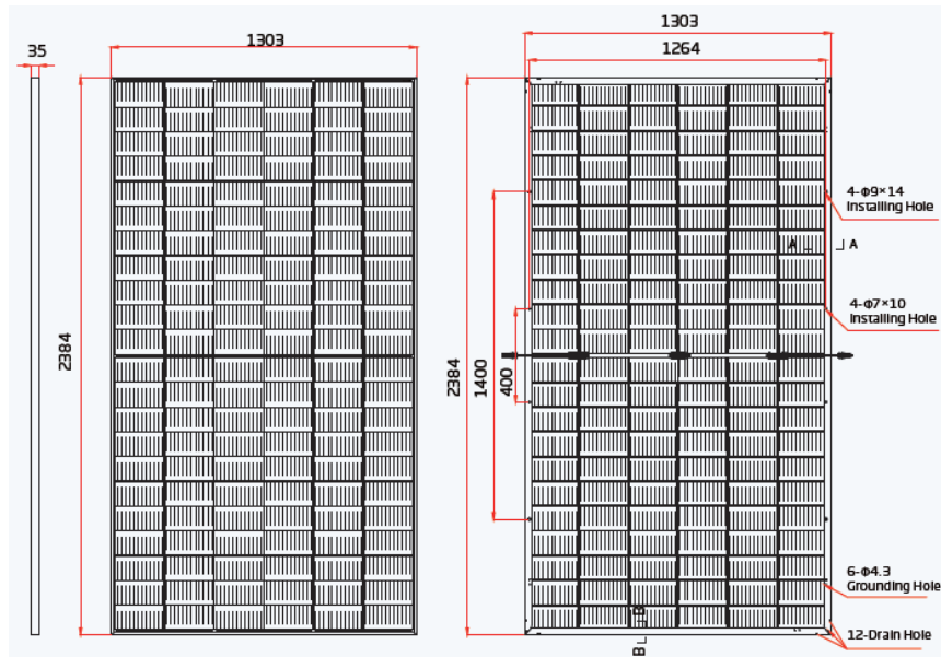
Figura 4.2.7.1.1.- Módulo fotovoltaico de proyecto (Fuente: Promotor)
