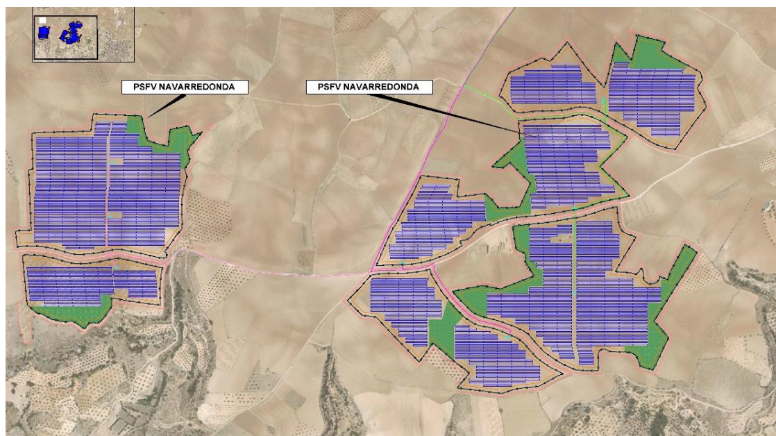
Figura 4.2.7.1.- Planta general de la PSFV.
