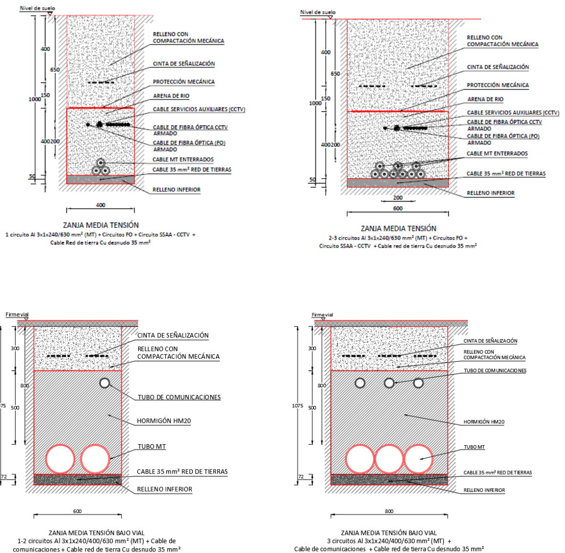
Figura 4.2.8.1.- Detalles de zanjas subterráneas previstas
