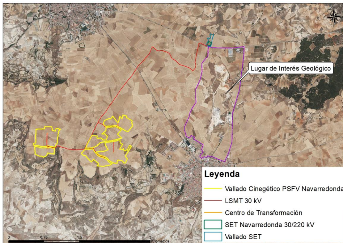
Figura 7.8.1. – Lugares de Interés Geológico (Fuente: IGME)
