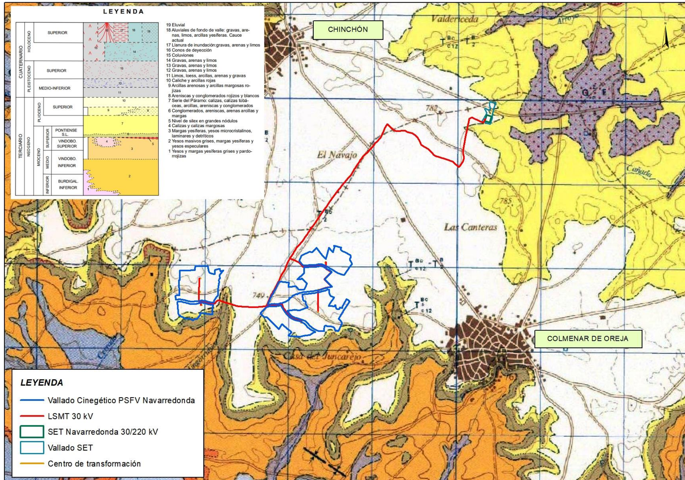
Figura 7.3.1.1 - Mapa geológico (Fuente: MAGNA 50 . Hoja 606)
