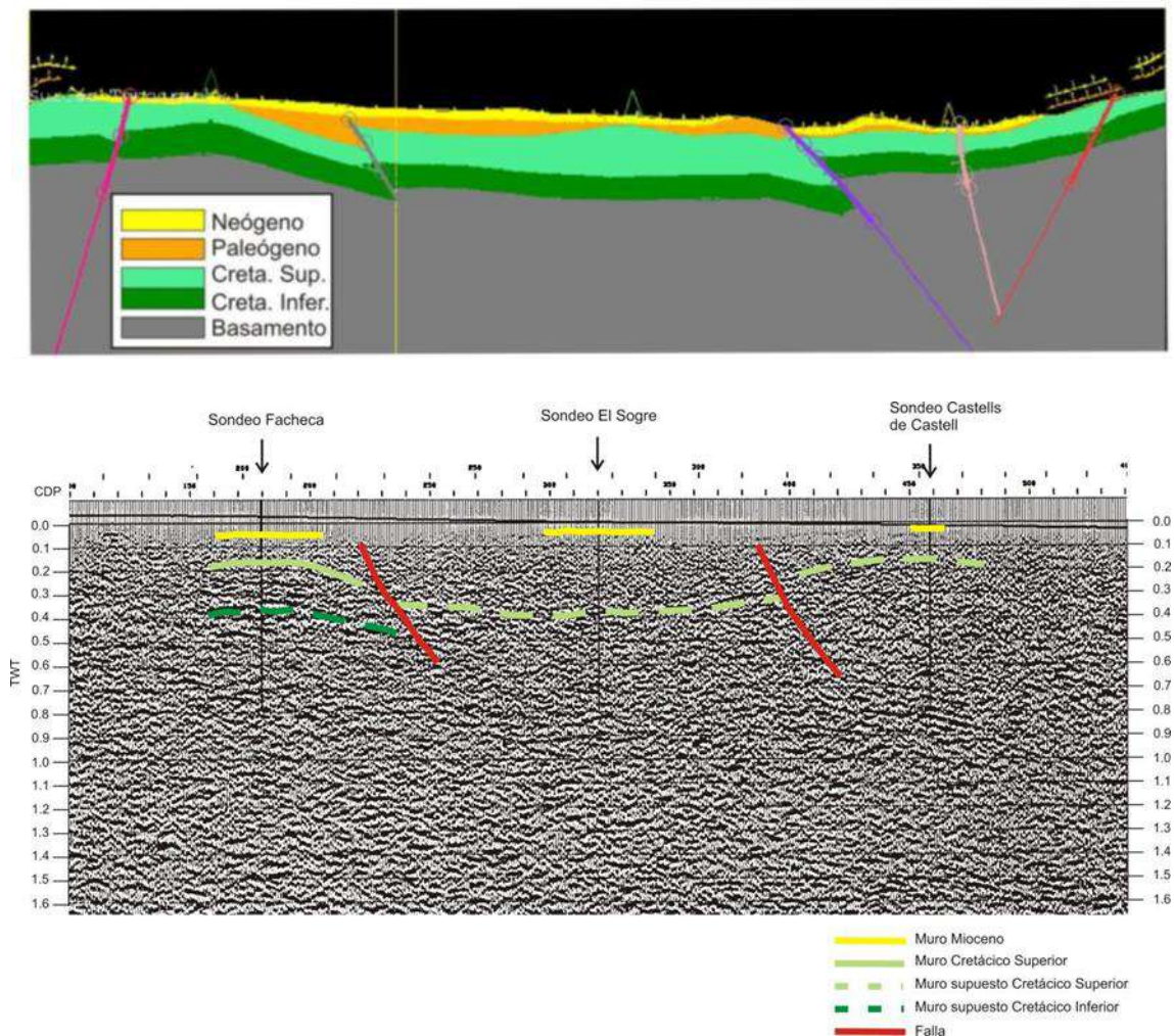
Figura 7. Línea sísmica RV-71V interpretada a partir de los sondeos Facheca, El Sogre y Castell de Castells. Acuífero Mediodía. Línea sísmica y corte 8 se posicionan en la figura 9B (el acuífero principal es el Cretácico Superior).
