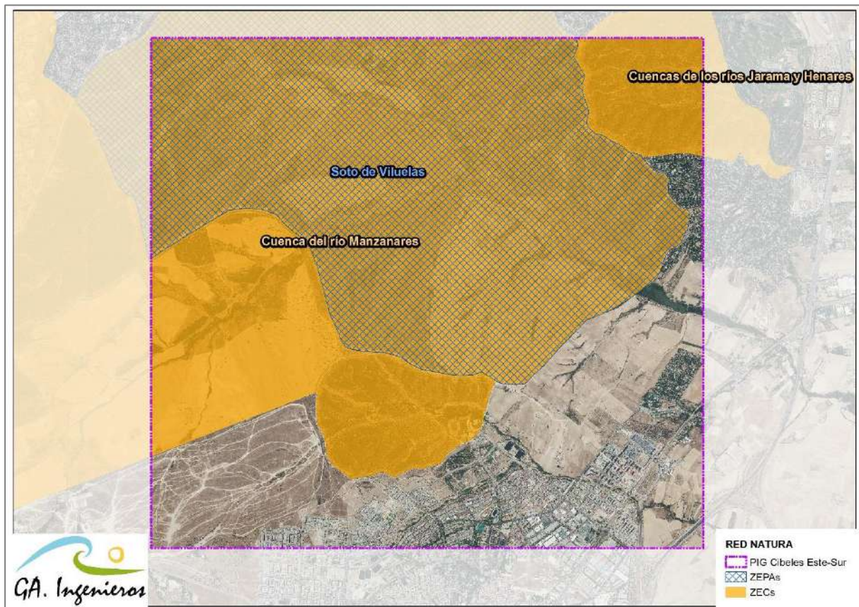
Figura 22. Red natural de Madrid con respecto al Permiso de Investigación “Cibeles Este Sur”.
