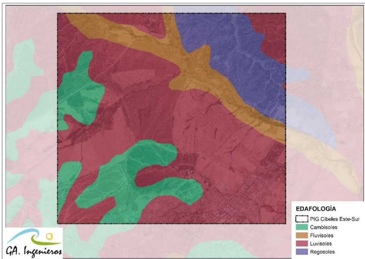
Figura 19. Edafología en el entorno de “Cibeles Este Sur”
