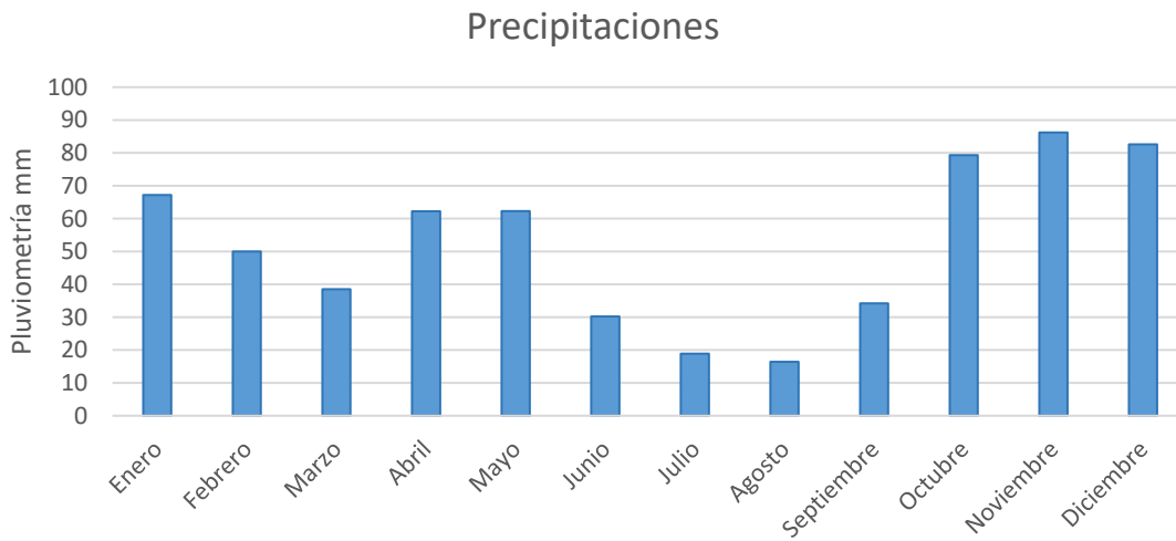
Gráfica 2. Distribución anual de las precipitaciones.
