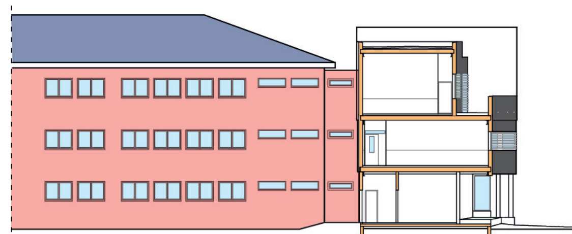
Sección B-B
